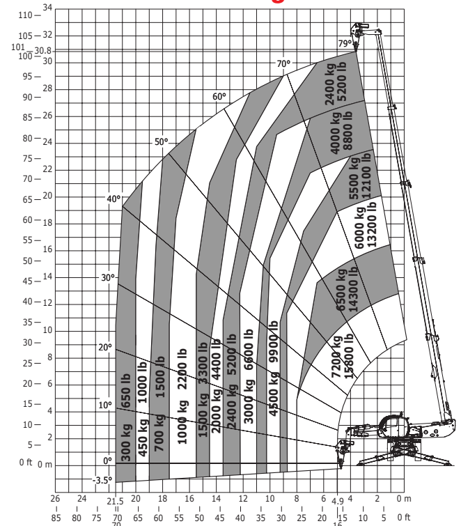
Rotation sur stabilisateurs déployés avec treuil 7200 kg
