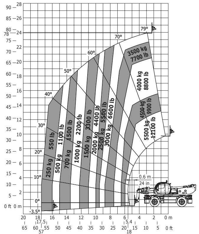
Frontal sur pneus avec fourches
